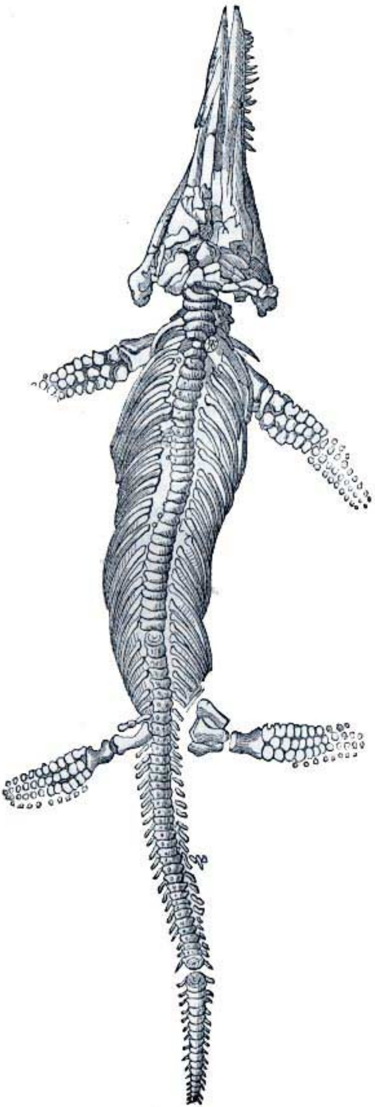
96.— Ichthyosaurus platydon .
